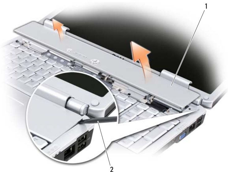
1 scharnierkap 2 pennetje
