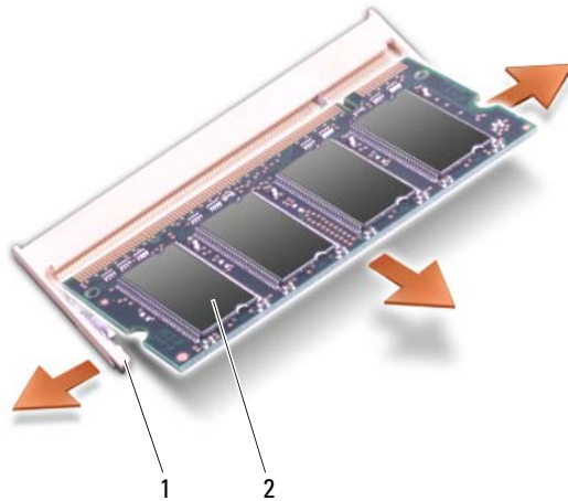
1 bevestigingsklemmen (2) 2 geheugenmodule
